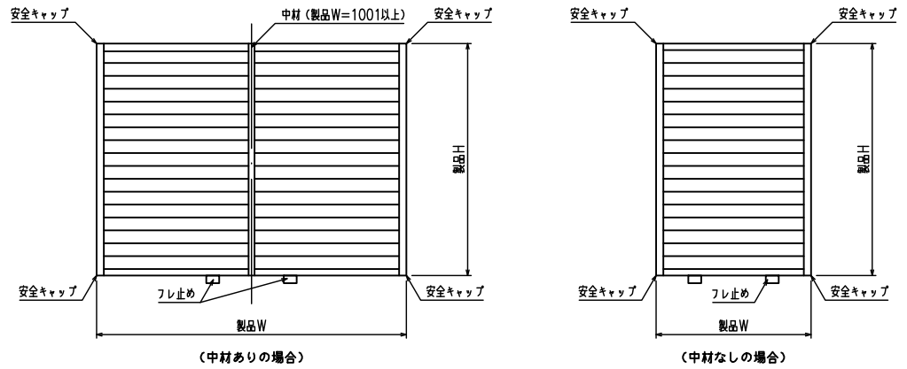
外觀図
