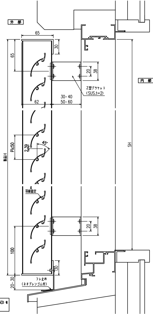
縦断面図
