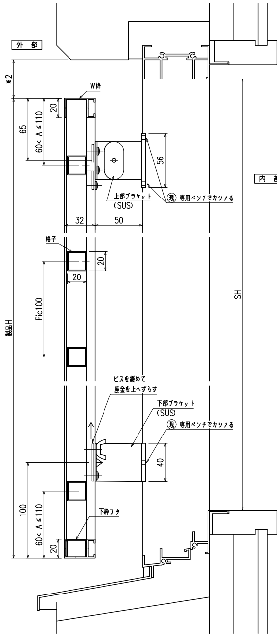
縦断面図
