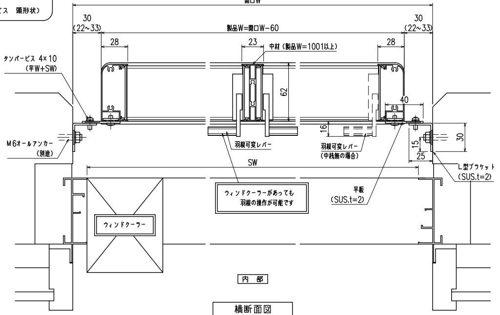
横断面図
