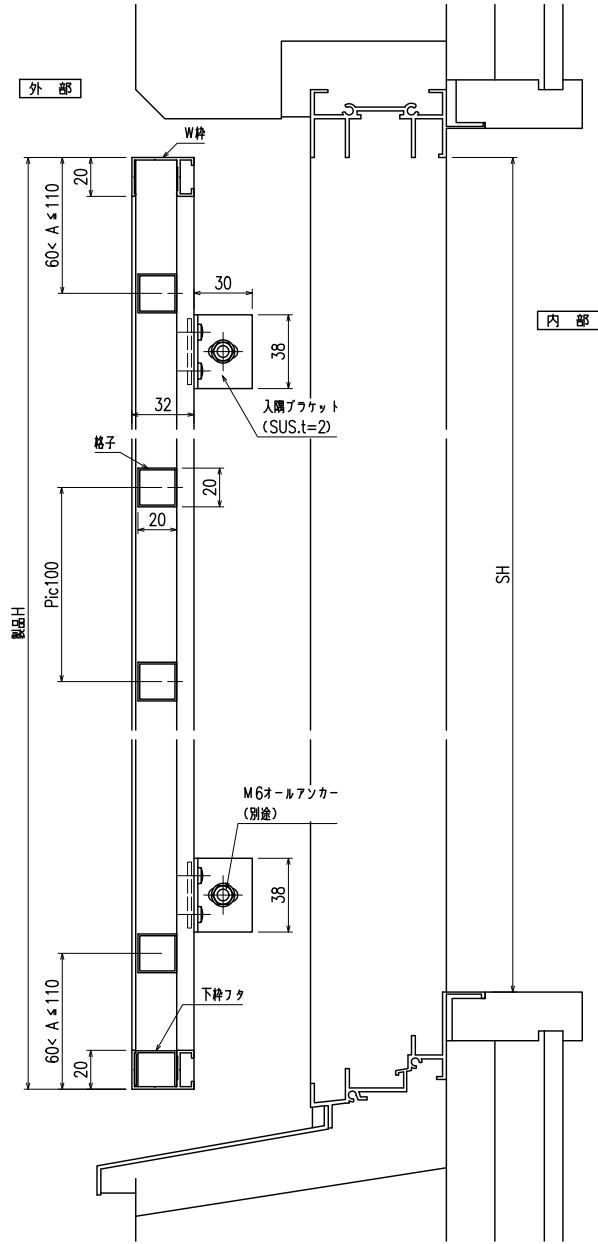
縦断面図
