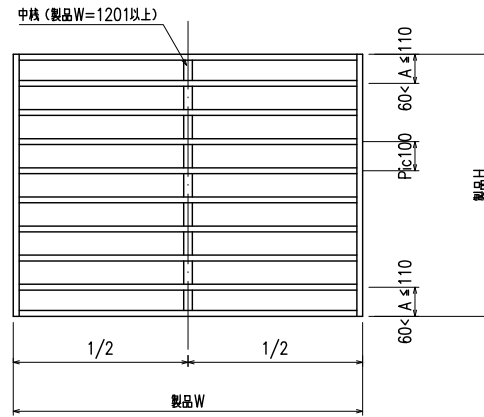
外観姿図
