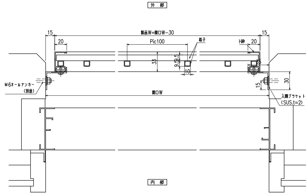
横断面図
