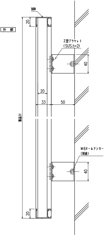
縦断面図
