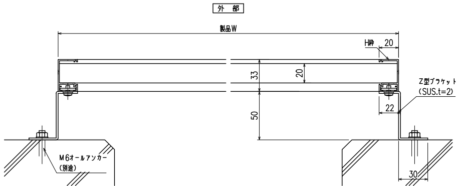
横断面図
