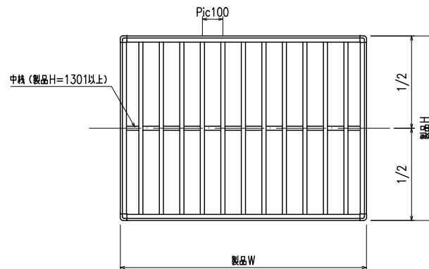
外観姿図
