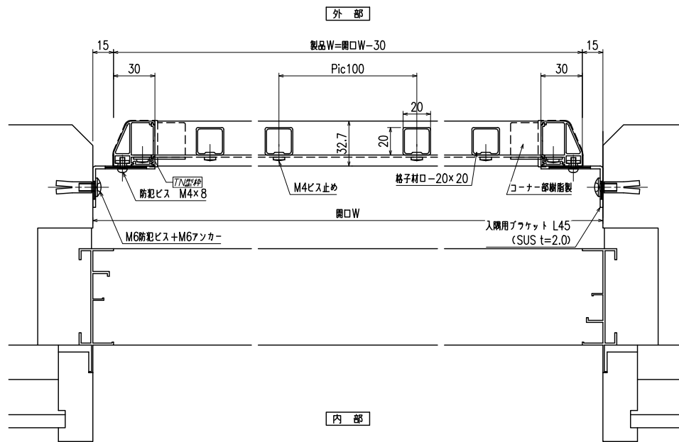
横断面図
