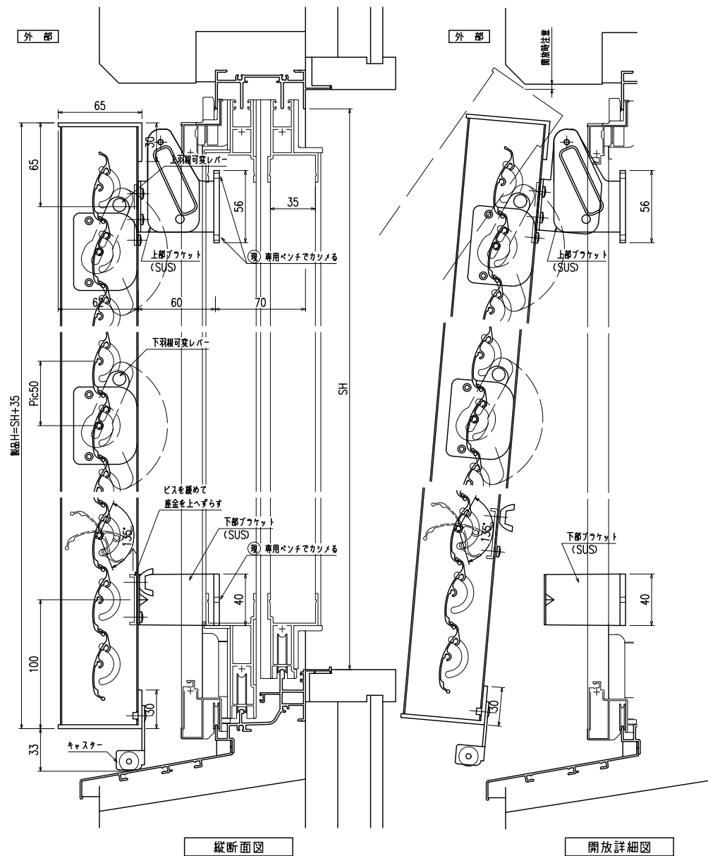
縦断面図
