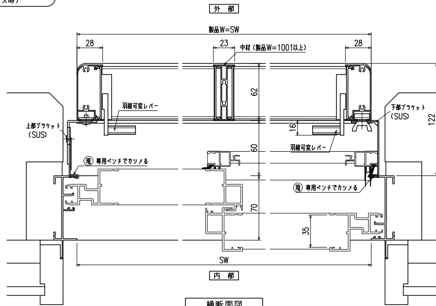
横断面図
