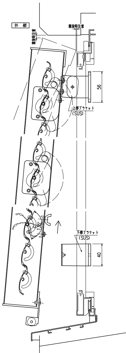
開放詳細図
