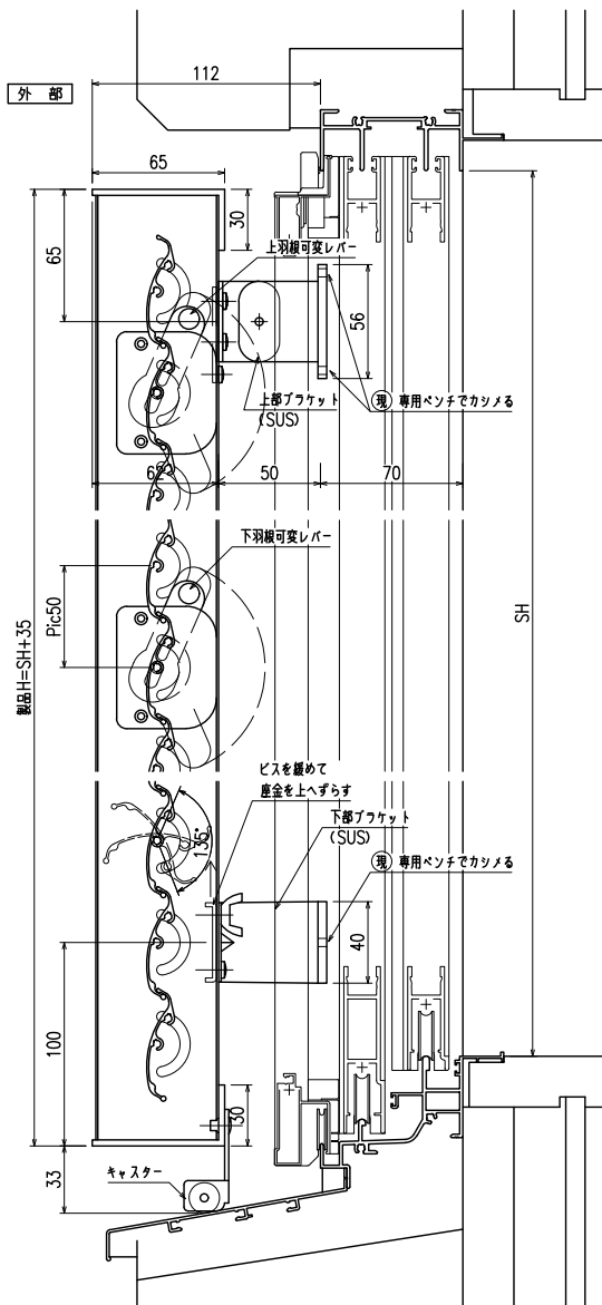
縦断面図
