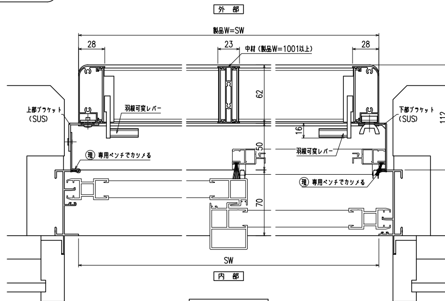
横断面図
