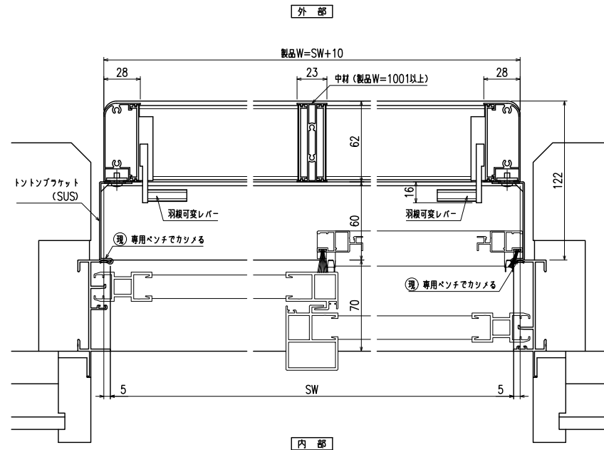
横断面図
