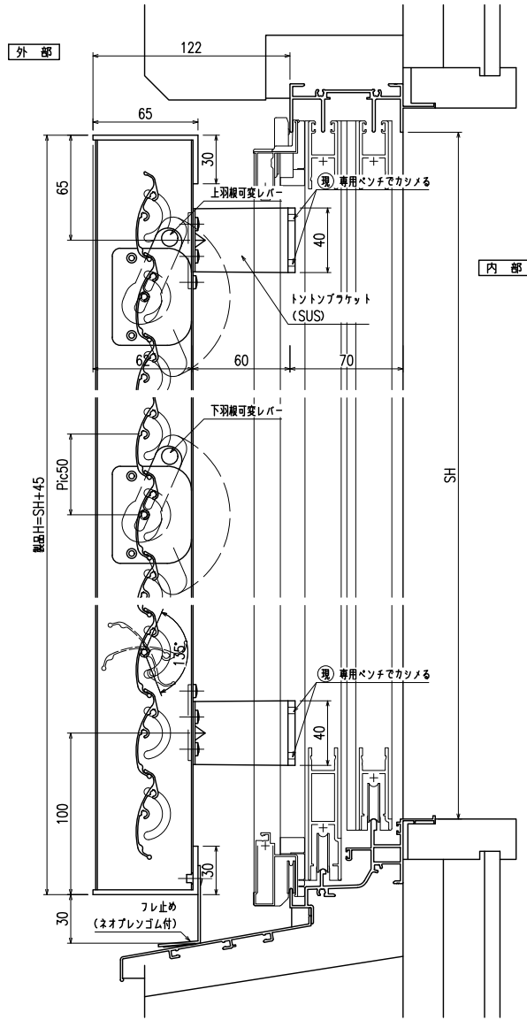
縦断面図
