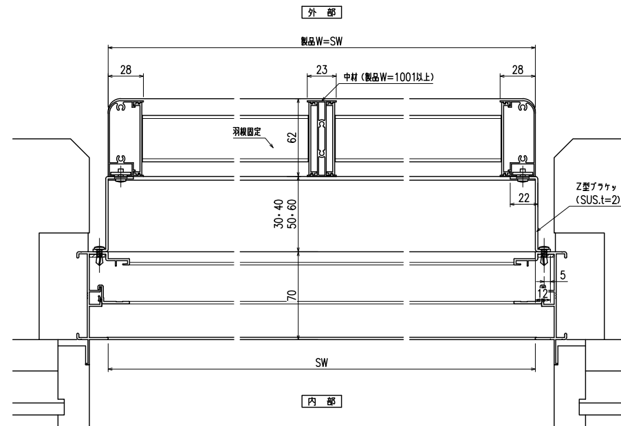
横断面図
