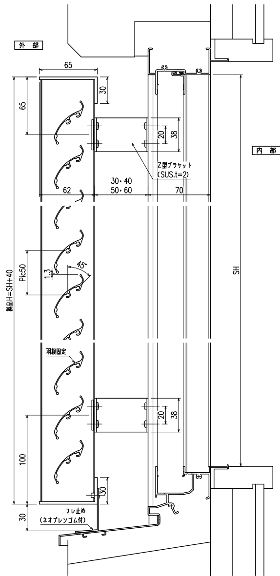
縦断面図
