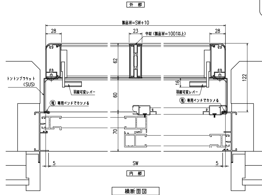
横断面図
