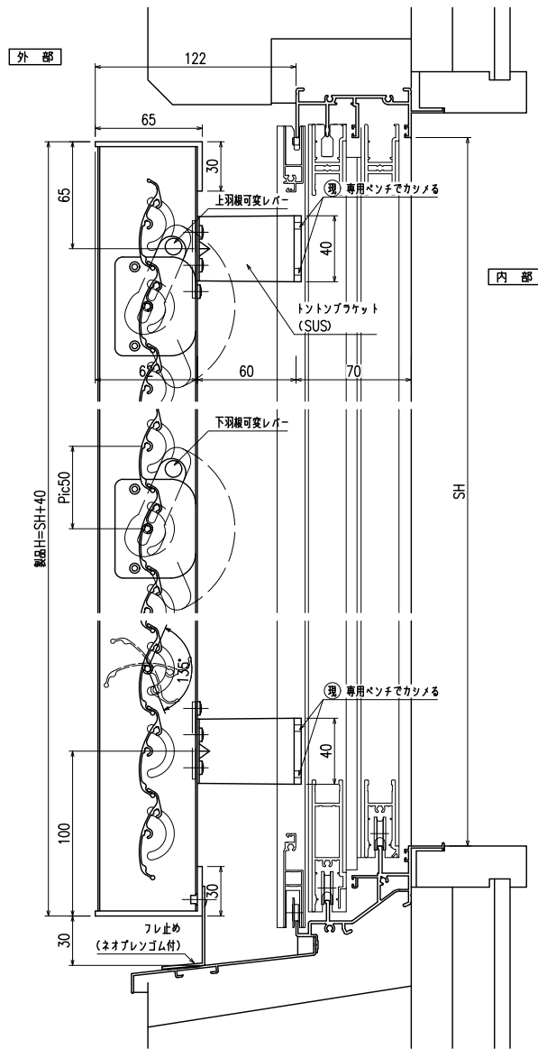
縦断面図
