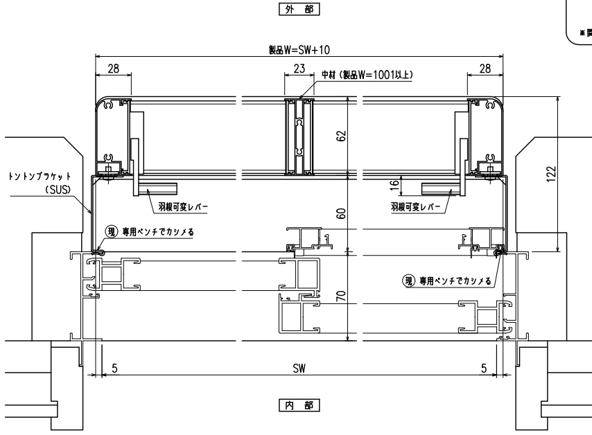
横断面図
