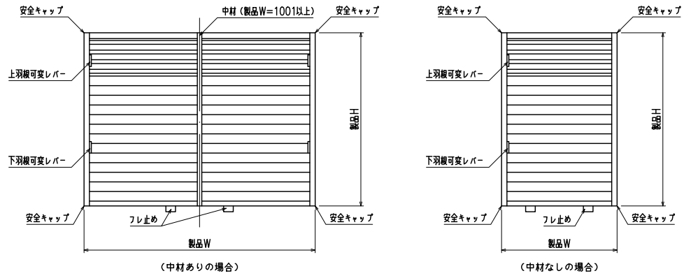
外観姿図
