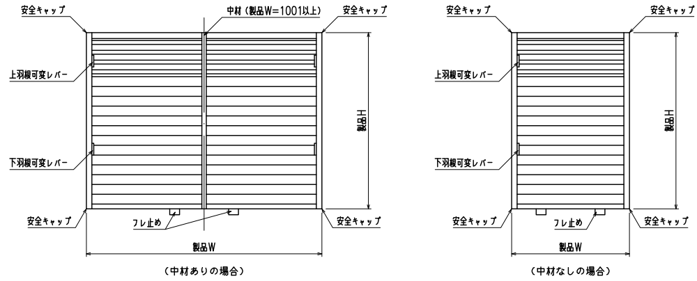
外觀姿図
