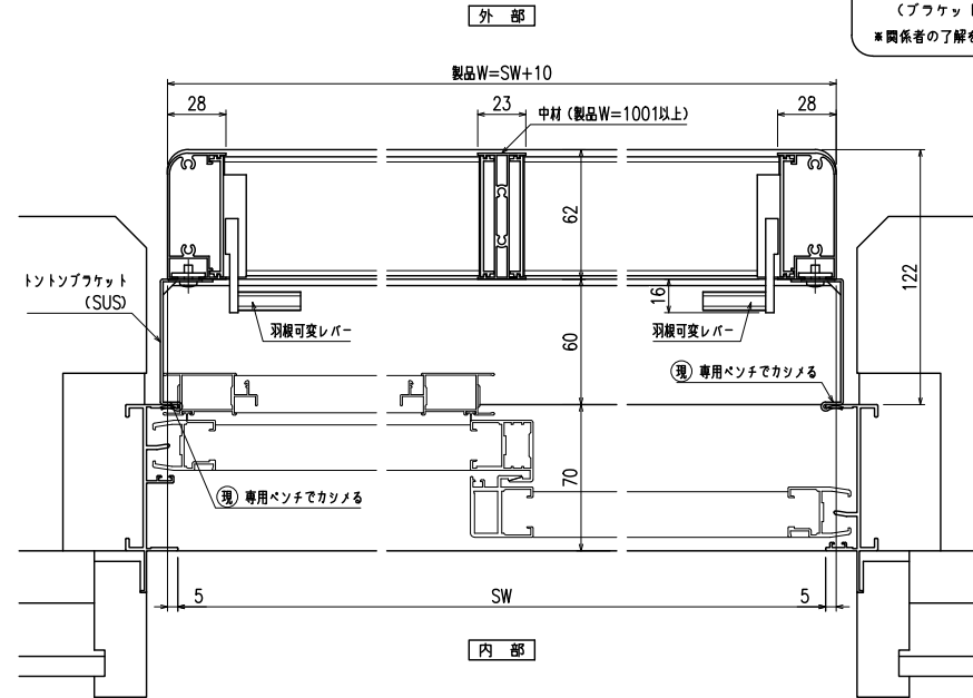
横断面図
