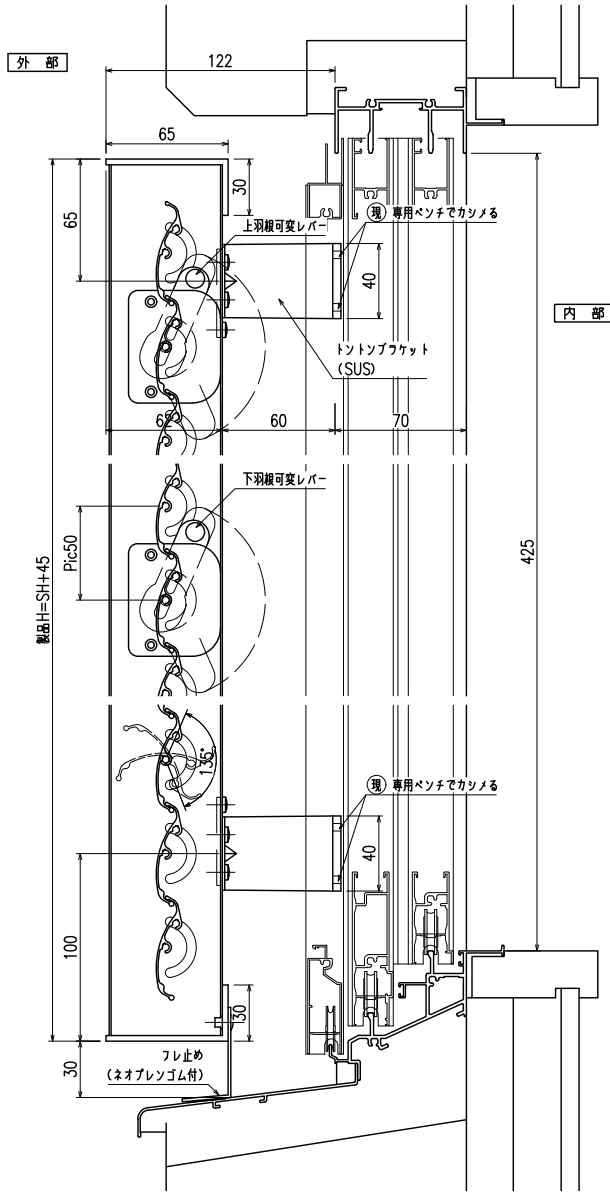
縦断面図
