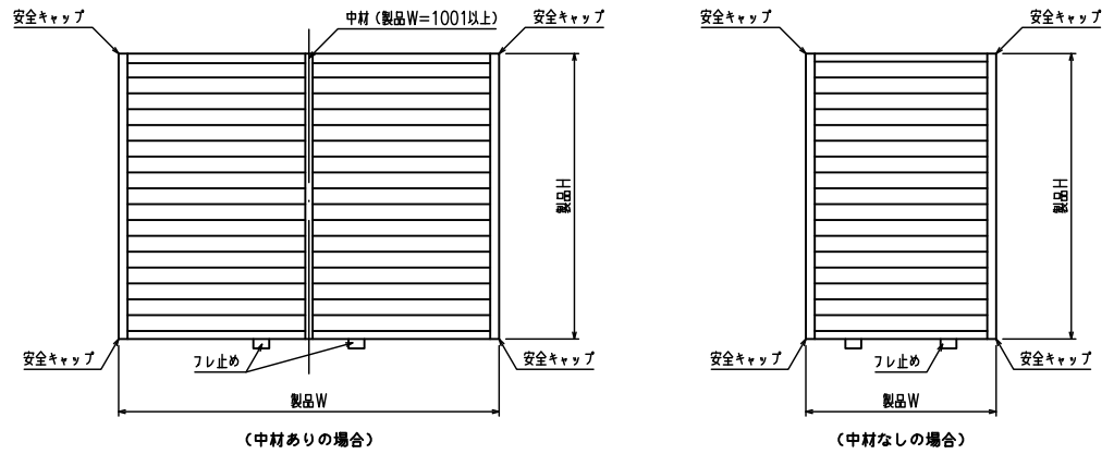
外観図
