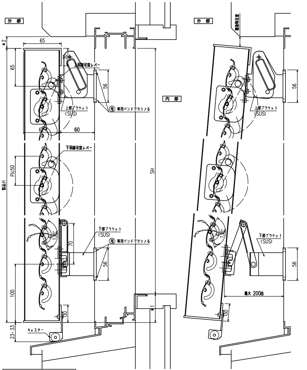
縦断面図
