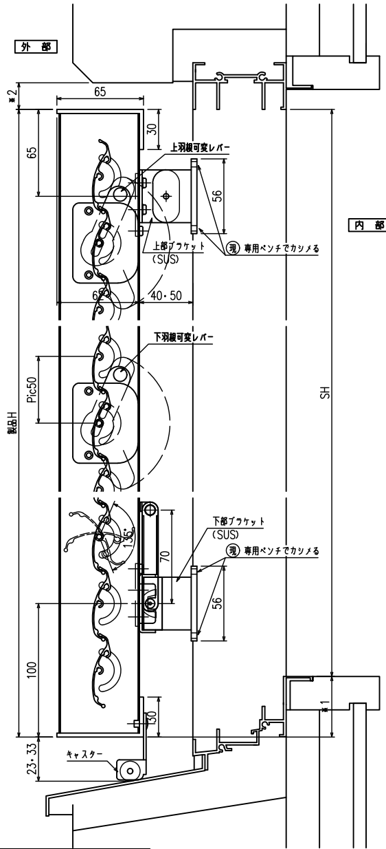
縦断面図
