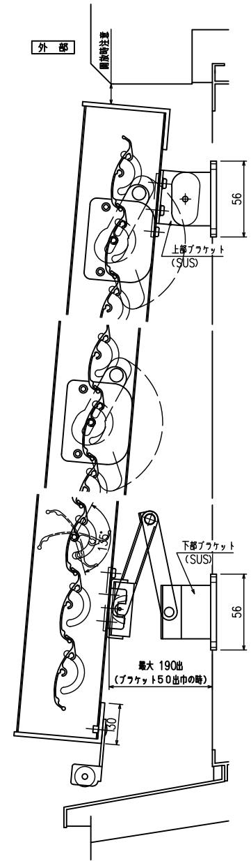
開放詳細図
