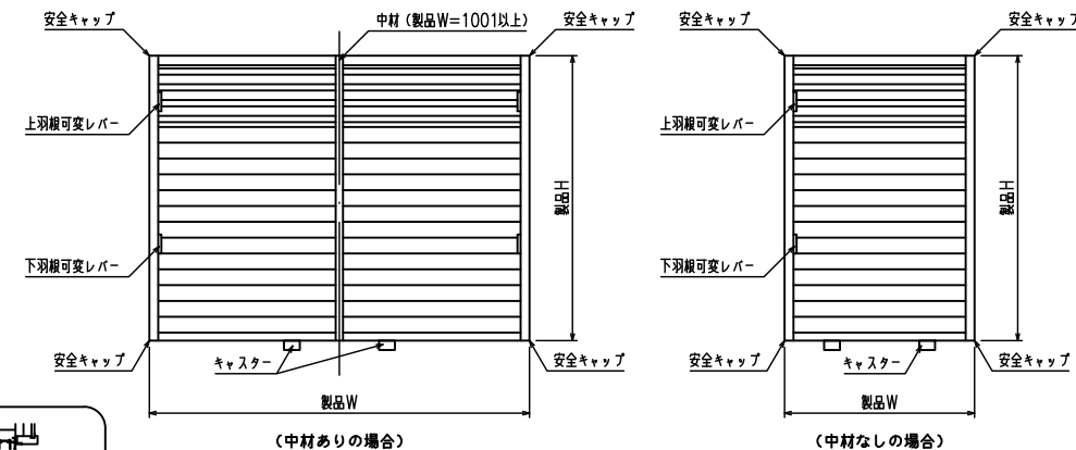
外観姿図
