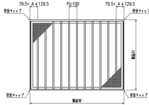
外観姿図
