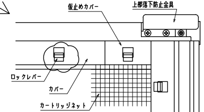
内観詳細図
