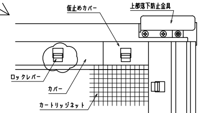
内観詳細図
