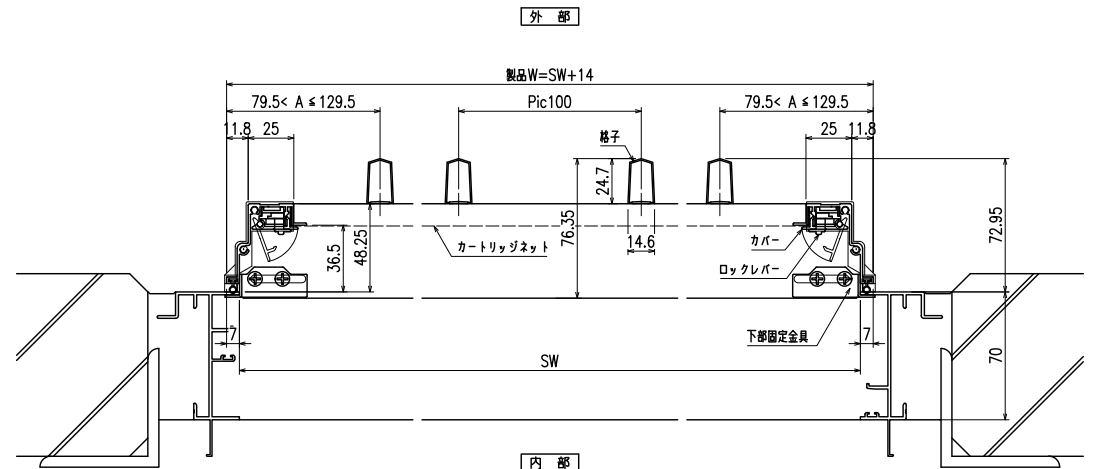
横断面図
