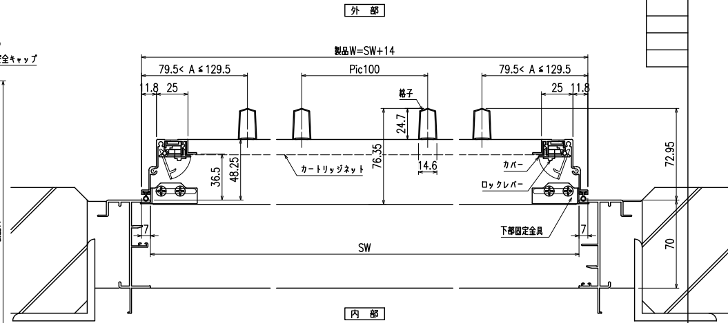
横断面図
