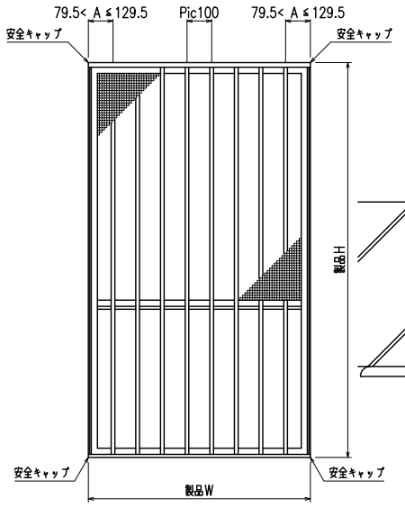
外観姿図
