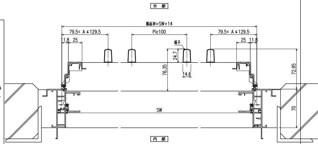
横断面図
