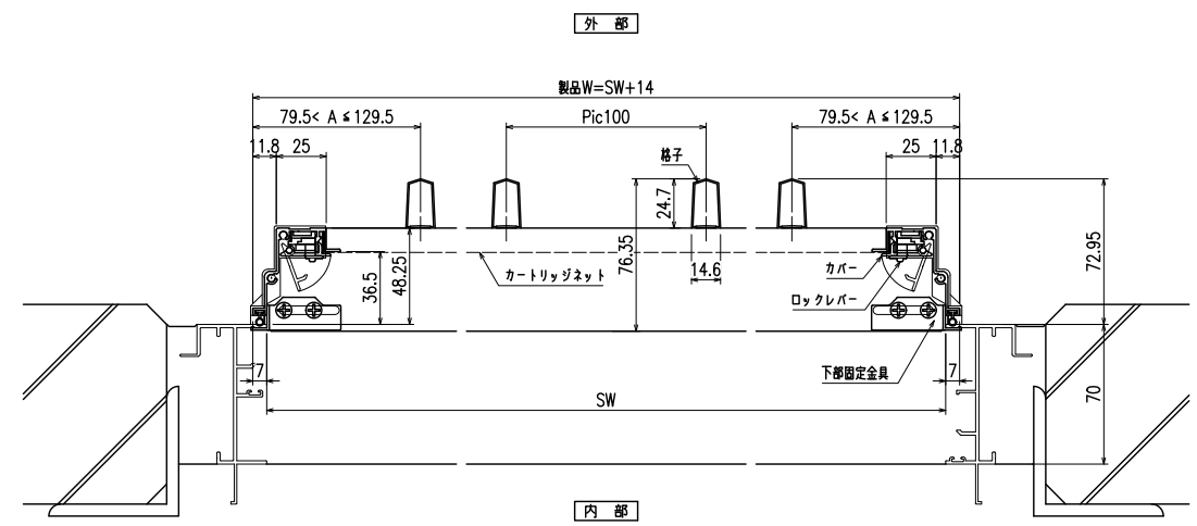
横断面図
