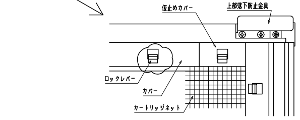
内観詳細図
