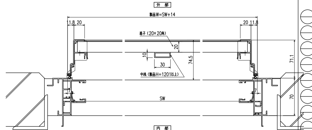
横断面図
