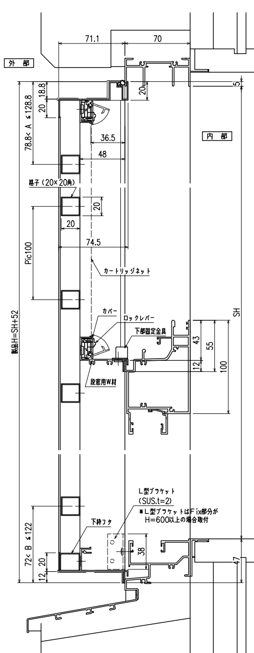
縦断面図
