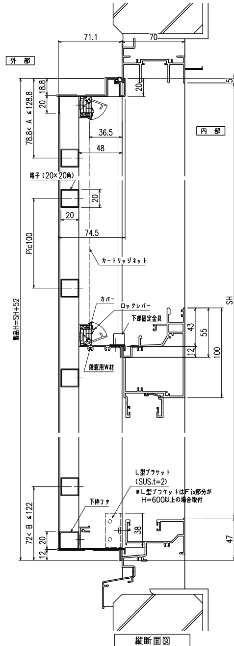
縦断面図
