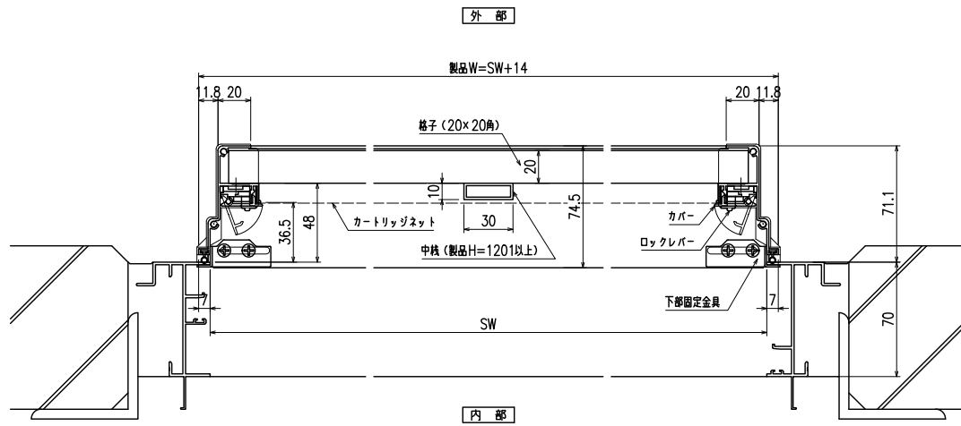
横断面図
