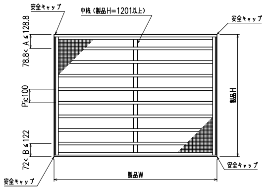
外觀姿図
