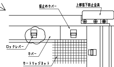
内観詳細図
