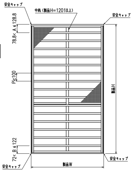
外觀図
