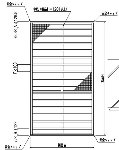
外觀姿図
