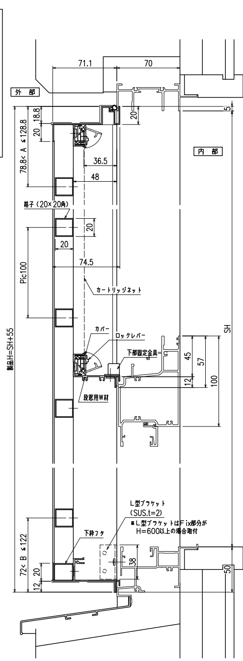
縦断面図
