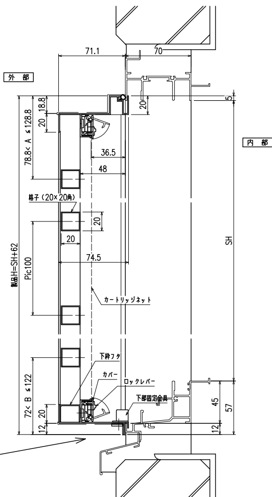
縦断面図
