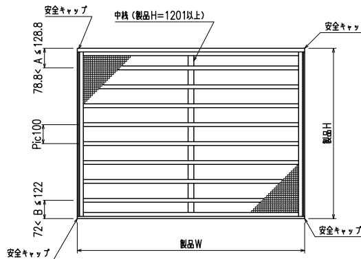
外観姿図
