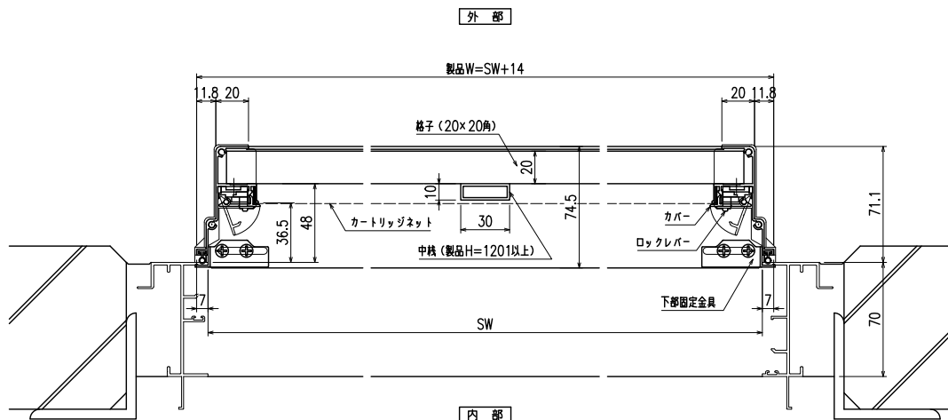
横断面図
