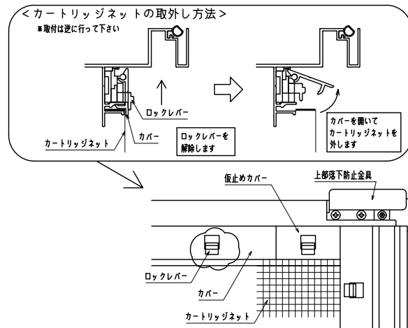
内観詳細図
