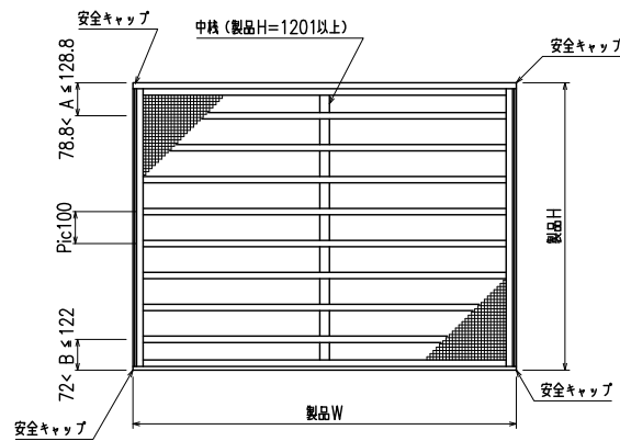
外観姿図
