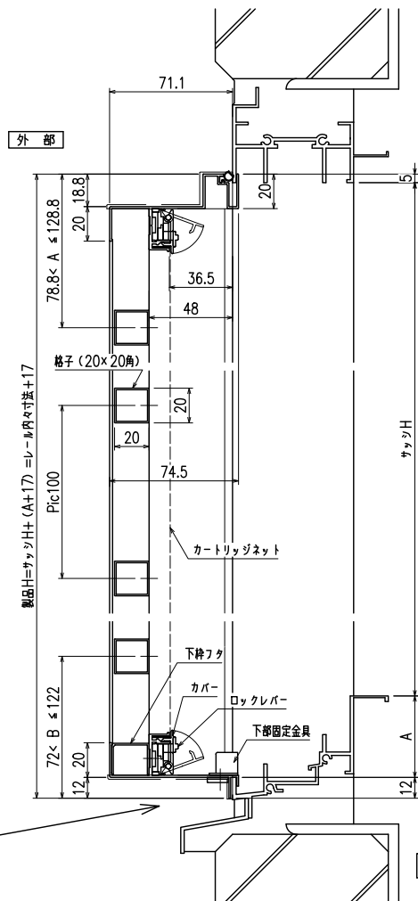
縦断面図
