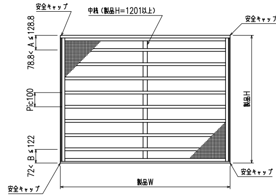
外観姿図
