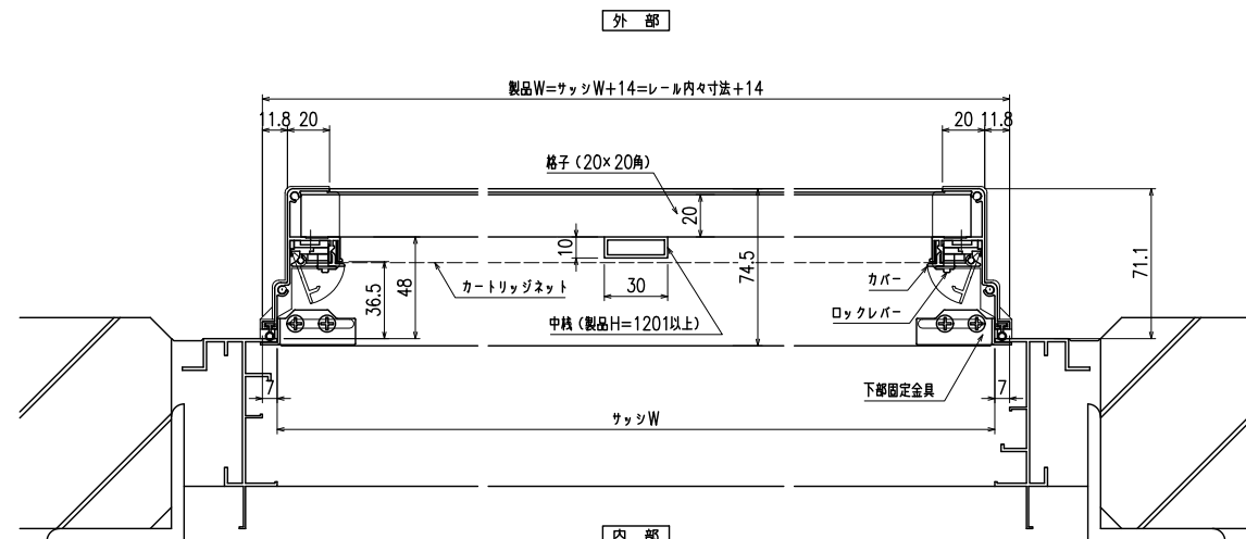
横断面図
