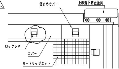
内観詳細図
