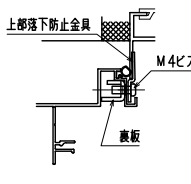
上部落下防止金具部分
