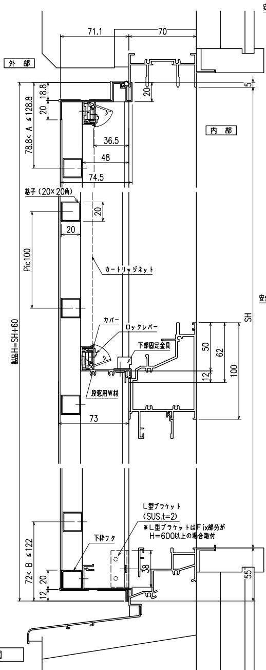
上部躯体のスキマ寸法について
