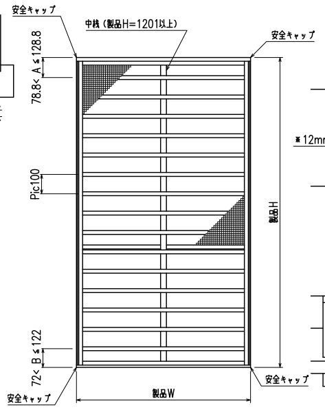
外観姿図
