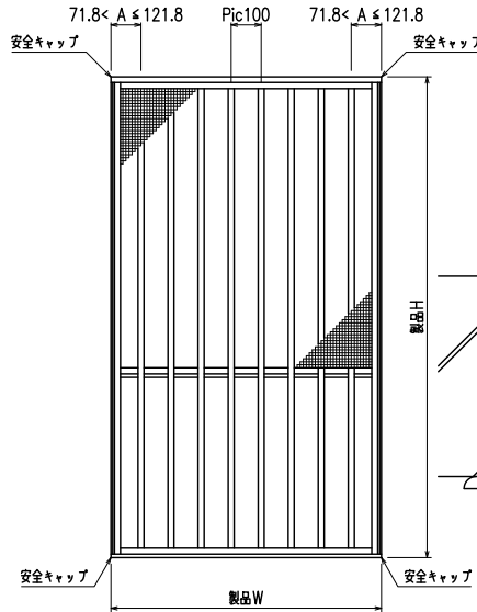
外観図
