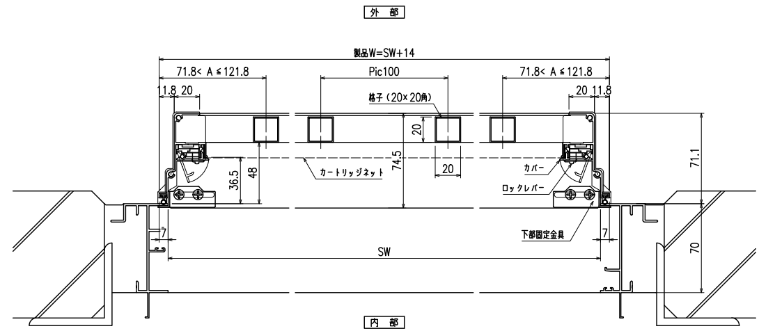
横断面図
