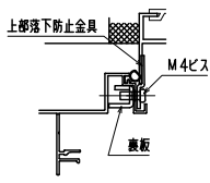
上部落下防止金具部分
