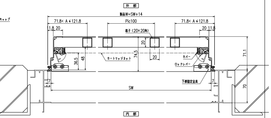
横断面図 (引き違い部分)
