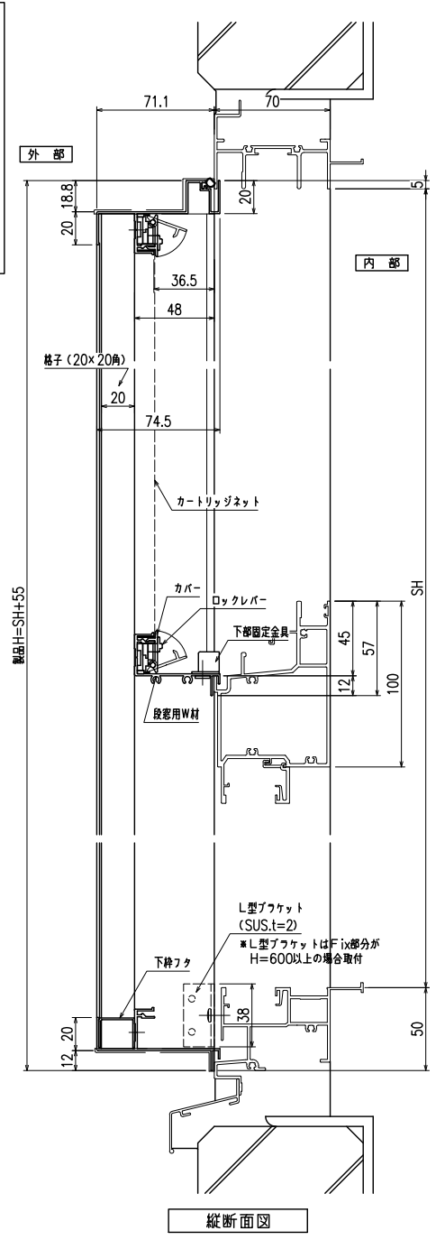
上部躯体のスキマ寸法について
