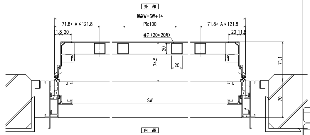
横断面図 (F1x部分)
