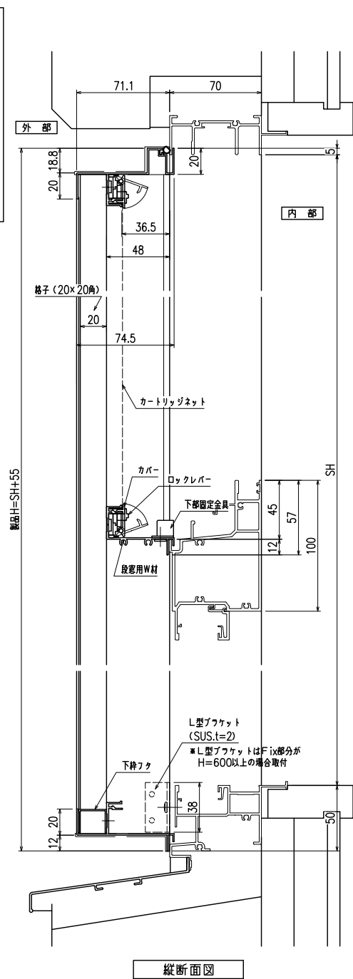
上部躯体のスキマ寸法について
