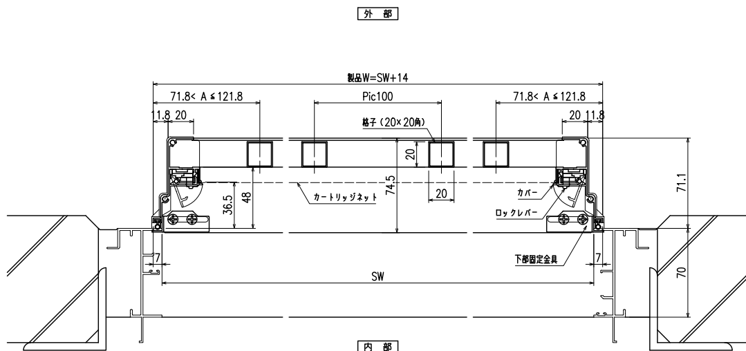
横断面図
