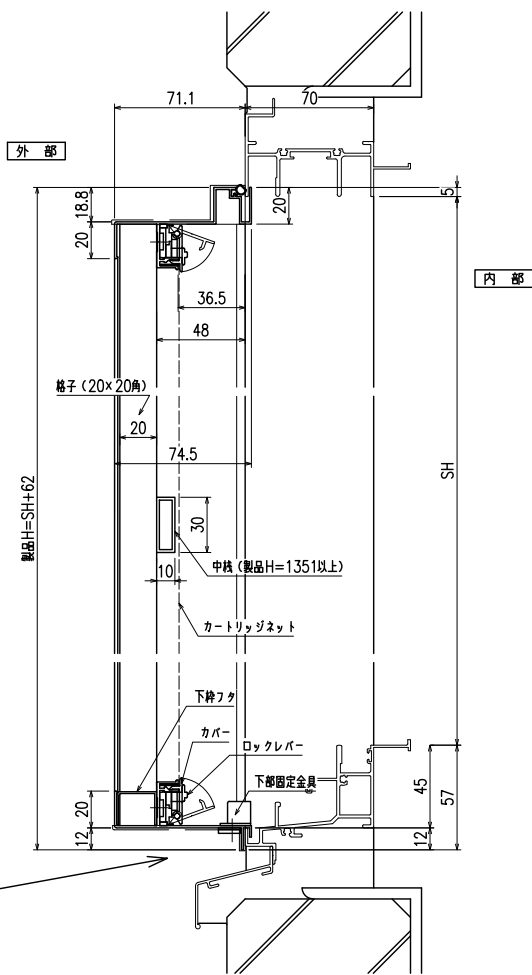
縦断面図
