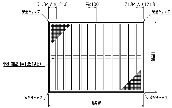
外観姿図
