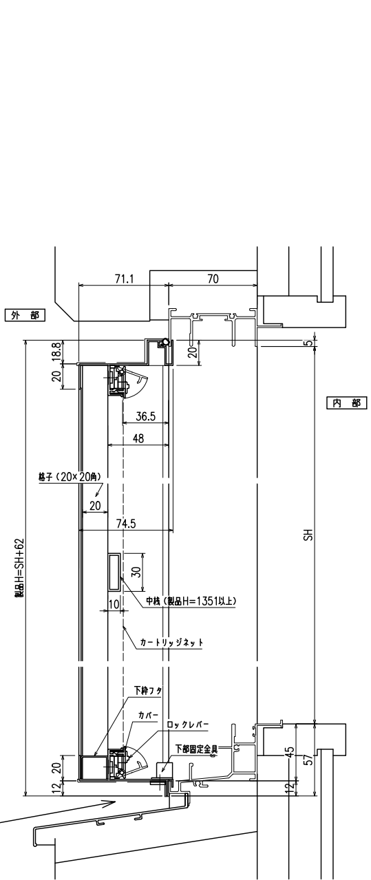
縦断面図
