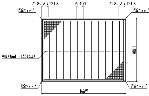
外観姿図
