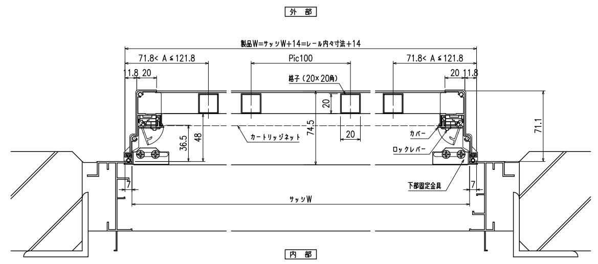
横断面図
