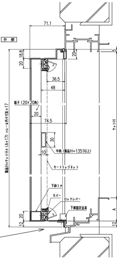
縦断面図
