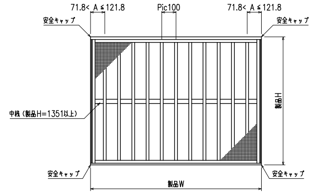
外観姿図
