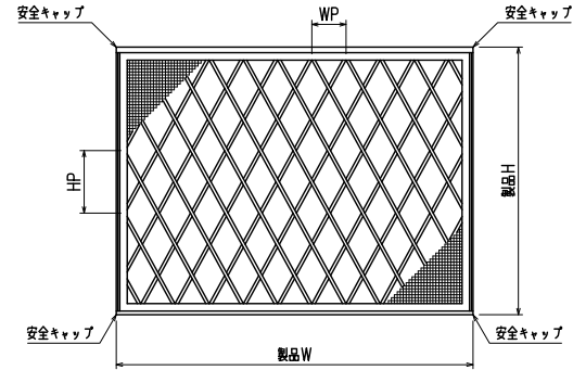
外観姿図
