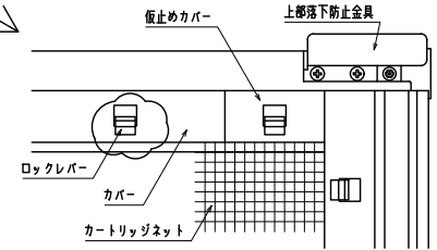
内観詳細図
