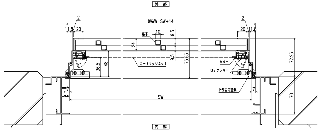
横断面図
