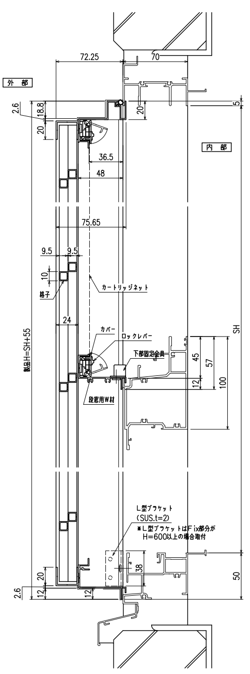
縦断面図
