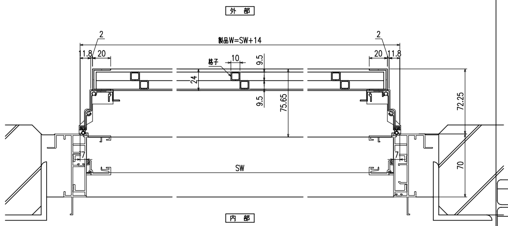
横断面図
