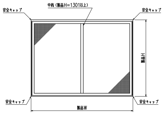
外観姿図
