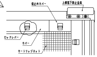
内観詳細図
