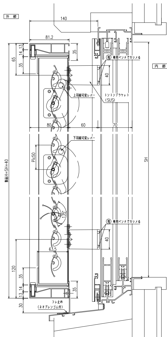
縦断面図
