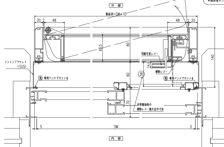
横断面図
