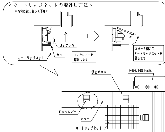
内観詳細図
