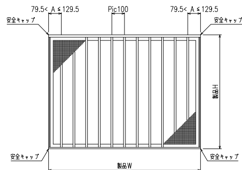
外観姿図
