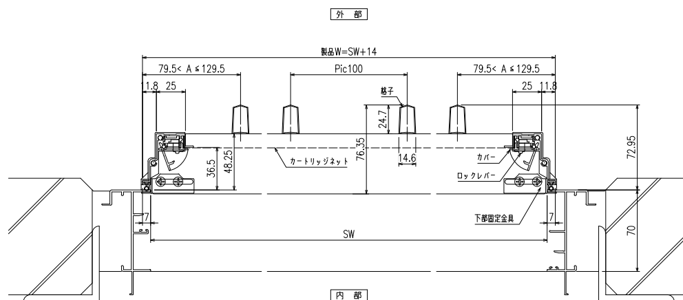
横断面図
