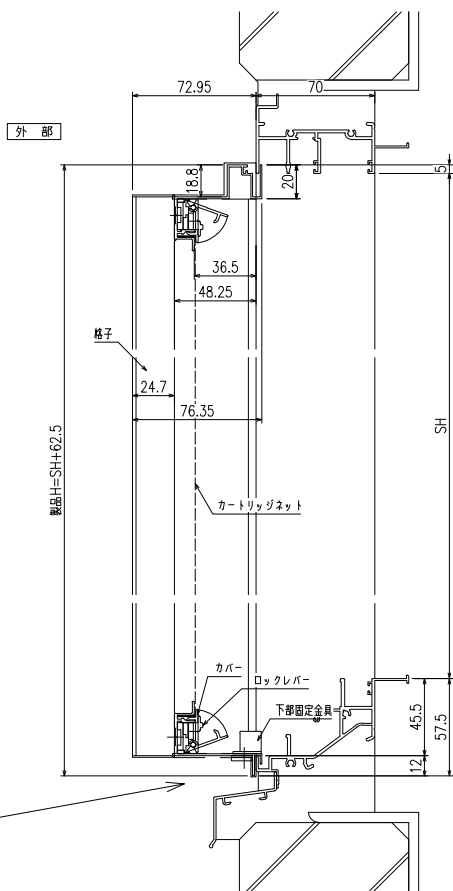
縦断面図
