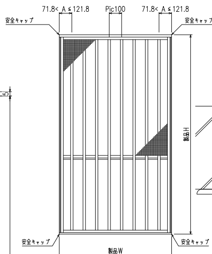
外観姿図
