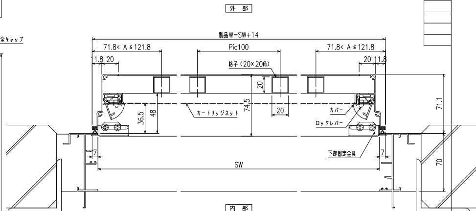
横断面図
