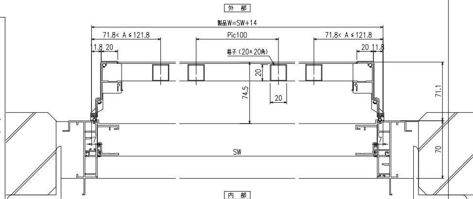
横断面図
