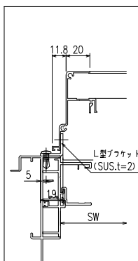
(L型ブラケット部分)
